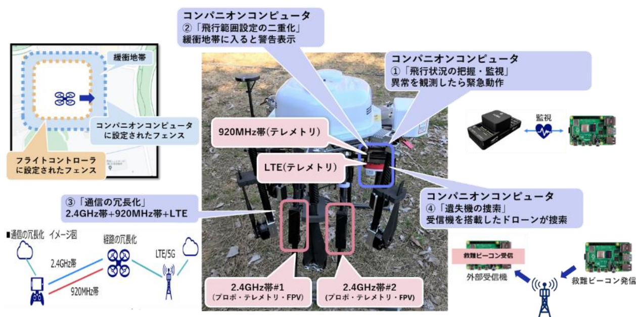
図 39 : 高可用性ドローン基盤開発事例
