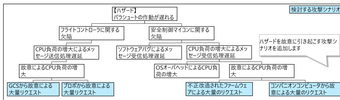
図 18 : パラシュートが開かなくなる故障を起こすための確認方法の例
