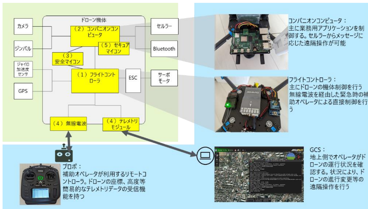
図 10：オープンソースドローンを構成するコンポーネント
