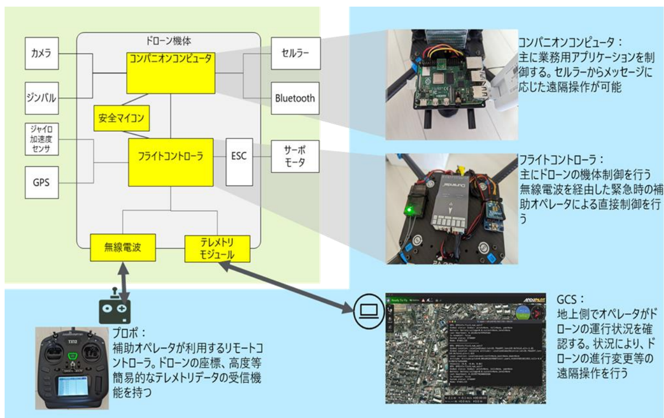
図 34：ドローン機体と周辺機器の構成
