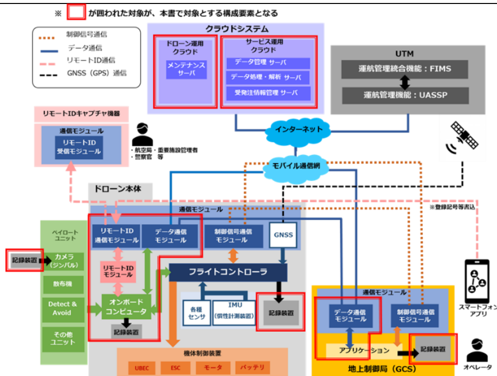
図 1 無人航空機の汎用的なシステムモデル（出典：経済産業省）
