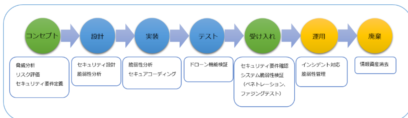
図 7 セキュリティ対策の全体的な流れ
